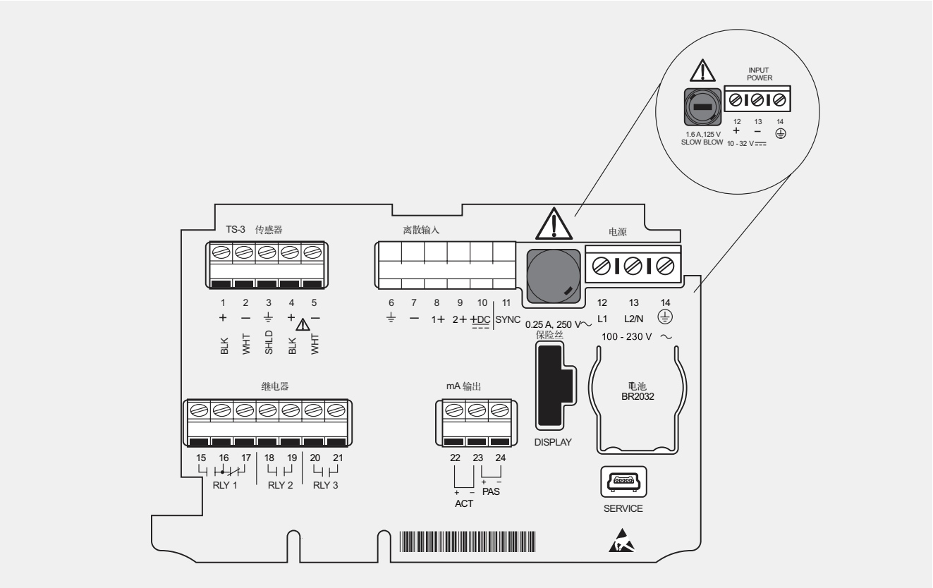
SITRANS LUT400 接线图
