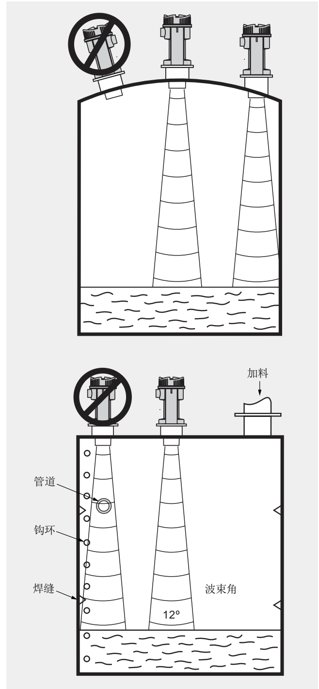
SITRANS LU180 的安装
