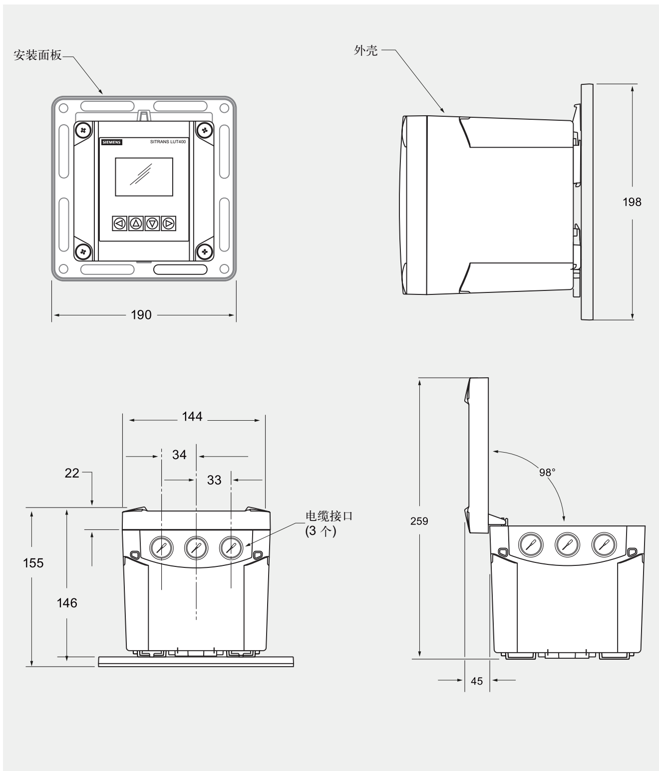
尺寸图
