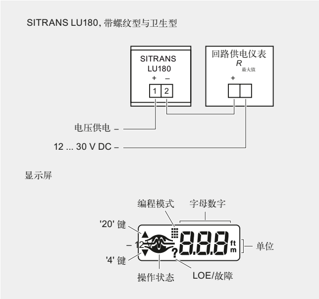
SITRANS LU180 的连接
