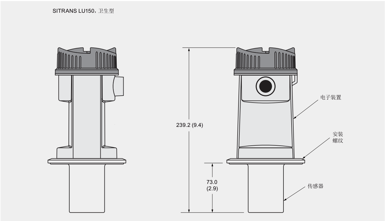
SITRANS LU150, 尺寸单位为 mm (英寸)
